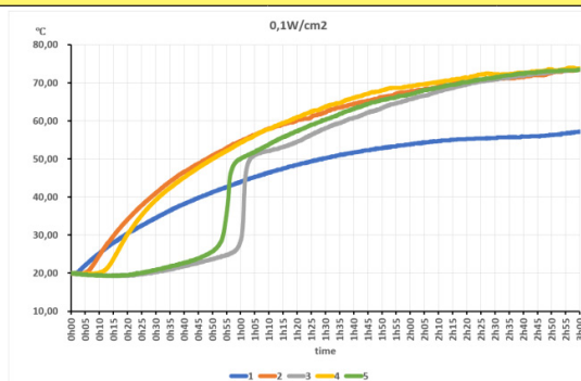
Bei einer Oberflächenlast von 0,1 W/cm 2 (60 W)
