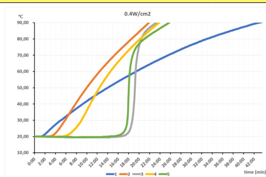
Bei einer Oberflächenlast von 0,4W/cm 2 (240W)
